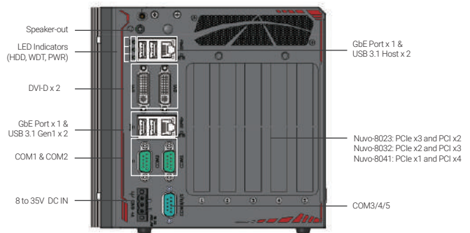
Nuvo-8023/ 8032/ 8041
